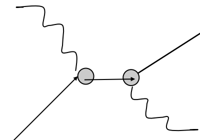
Σκέδαση Compton
