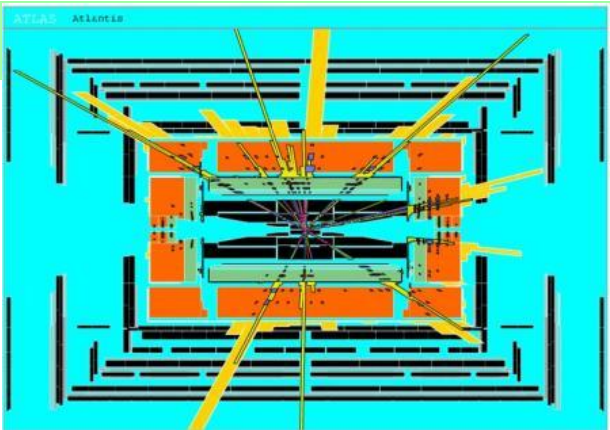
Από προσομοίωση: A mini-blackhole in ATLAS !
