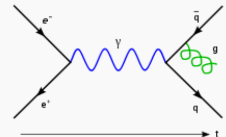
(Feynman diagram)
