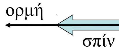
αντι -νεutrino
