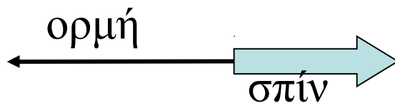
νεutrino
