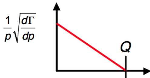
διάγραμμα Kurie.
