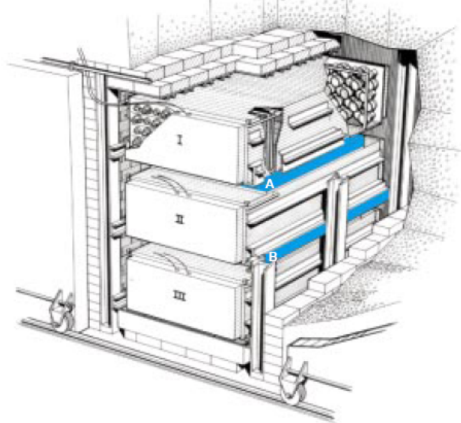
Διάταξη Reines – Cowan
