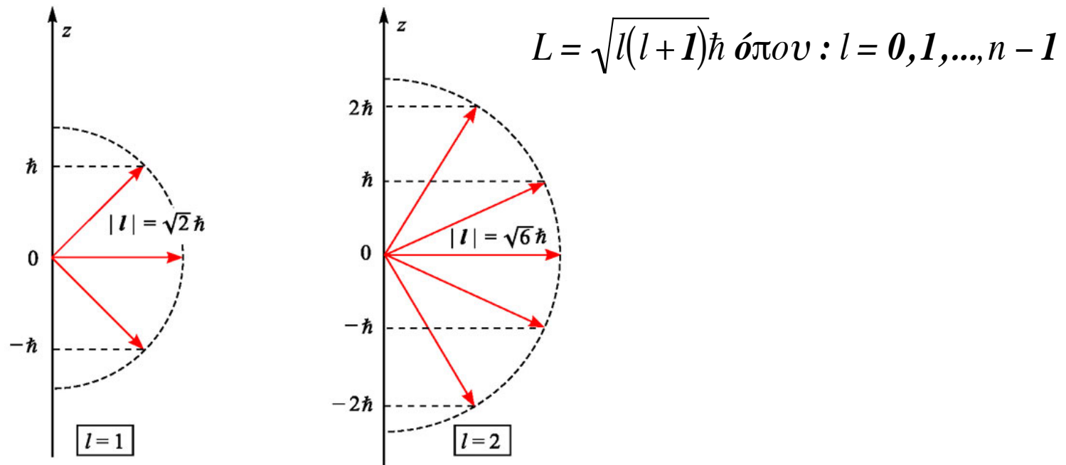
ΣΧΗΜΑ 9.9: Το κβαντωμένο διάνυσμα της στροφορμής για \ell = 1 και \ell = 2 . Λόγω της κβάντωσης της προβολής του πάνω σε έναν άξονα, το «διάνυσμα» της στροφορμής –αν η σχεδιάσή του ως διανύσματος έχει νόημα– μπορεί να έχει μόνο ορισμένους διακριτούς προσανατολισμούς στον χώρο. Φαινόμενο που αποδίδεται με τον όρο «κβάντωση προσανατολισμού» ή «κβάντωση χώρου». Σημειώστε επίσης –γιατί αυτό είναι το πιο προκλητικό από όλα– ότι το διάνυσμα \ell ουδέποτε ευθυγραμμίζεται με τον άξονα z . Ακόμα και στην κατάσταση μέγιστης προβολής του σε αυτόν τον άξονα σχηματίζει γωνία μαζί του αφού είναι πάντα (\ell_z)_{\max} = \hbar\ell < |\ell| = \hbar\sqrt{\ell(\ell+1)} .
